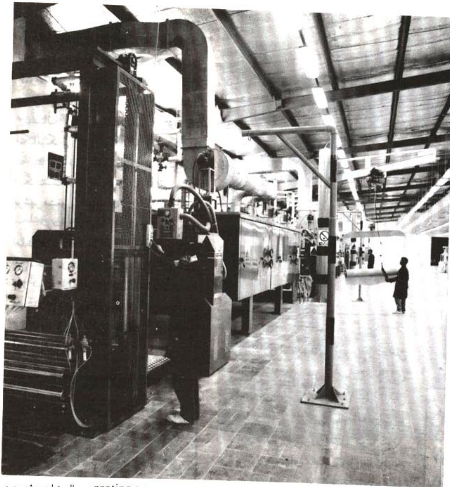
خط coating در سالن تولید پوشاک چرم
